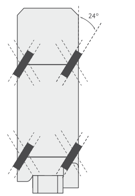
4 RUEDAS DIRECCIONALES CON MODO CANGREJO
