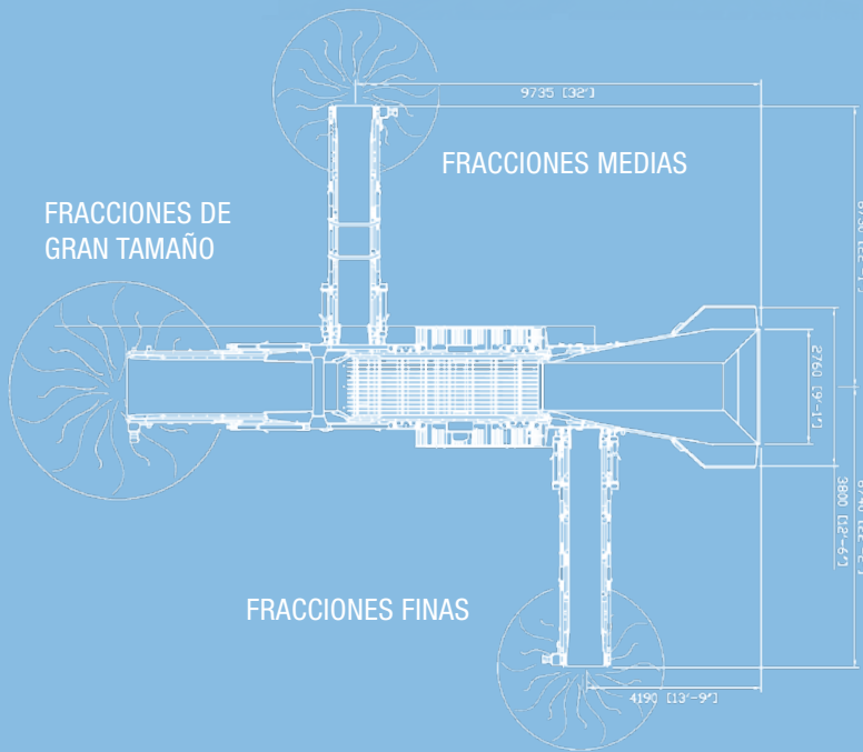
MOBISCREEN MS 15 Z VERSIÓN ESTÁNDAR
